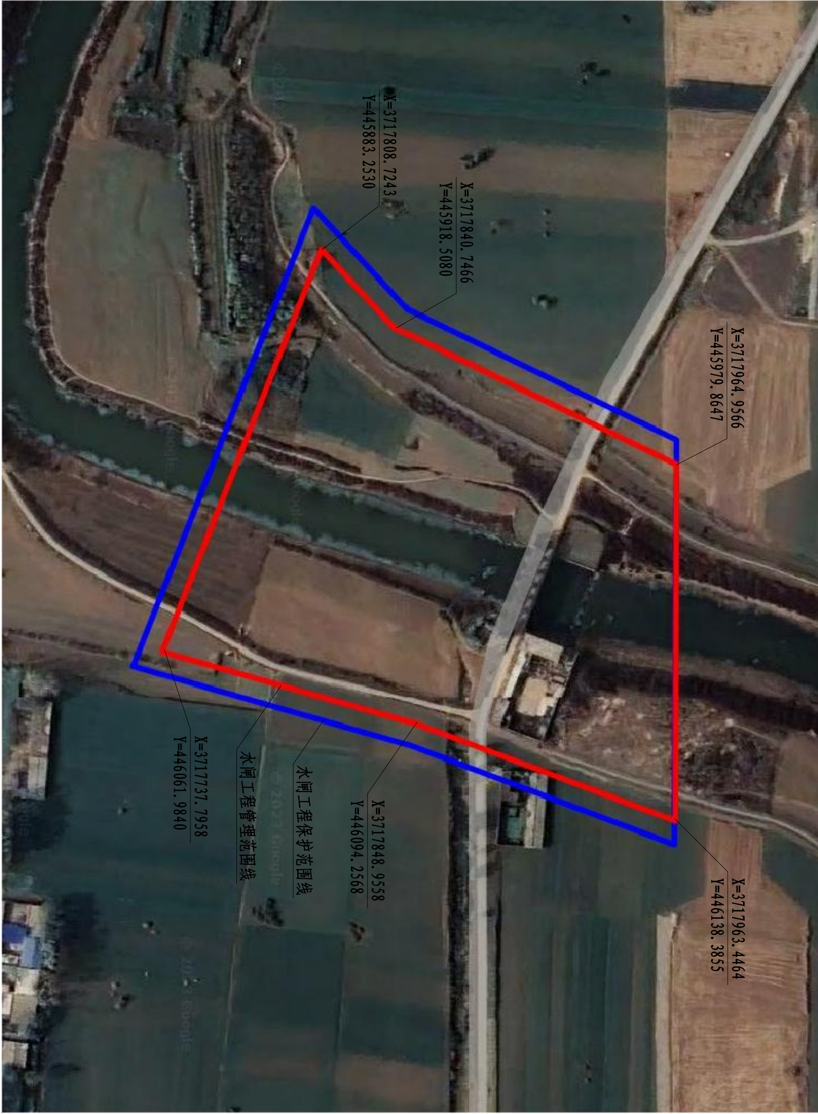
叶县灰河谷店闸管理与保护范围线图
